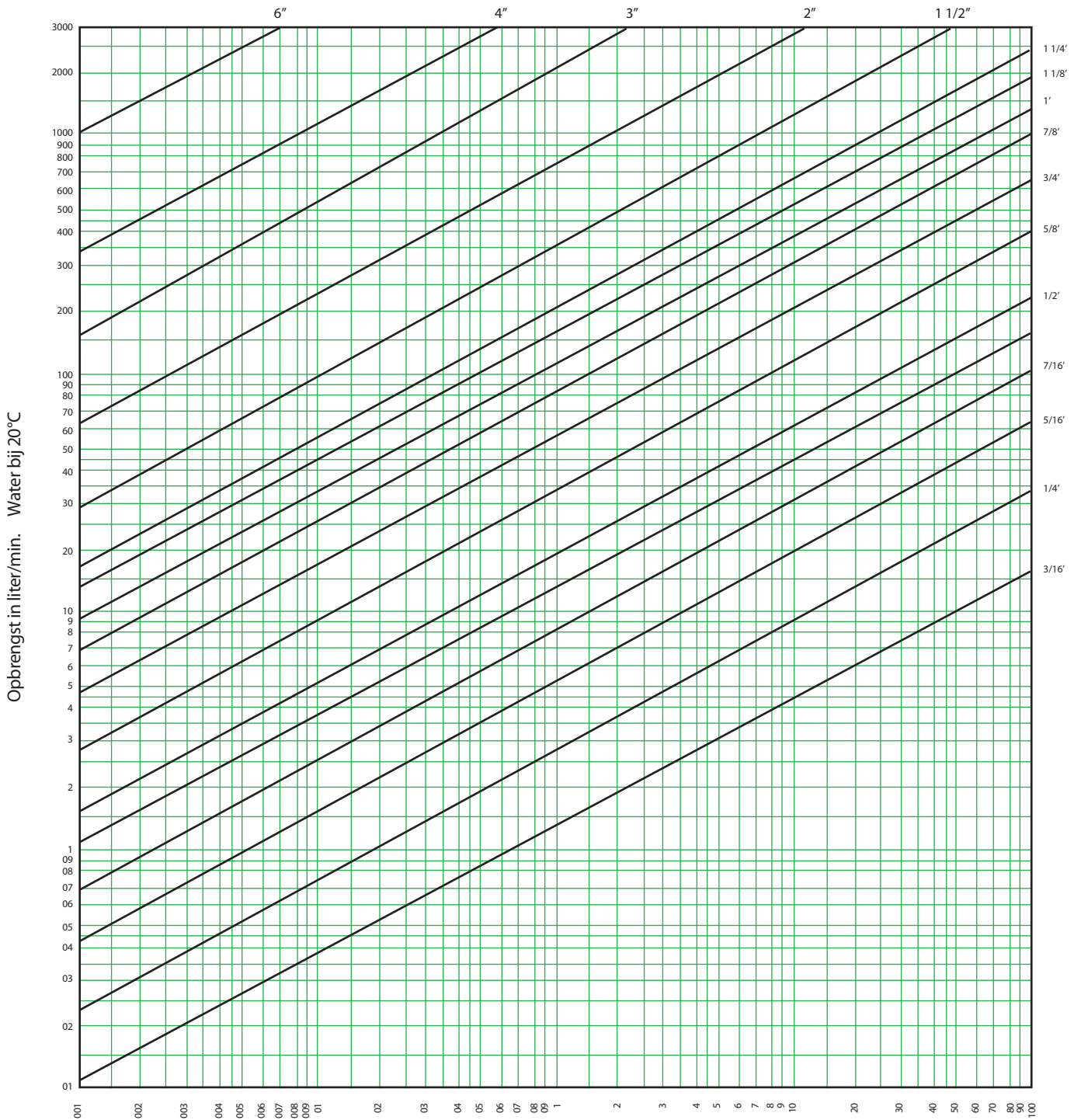
Drukverlies in bar bij een slanglente van 15 meter zonder koppelingen
